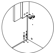
假门板安装图
